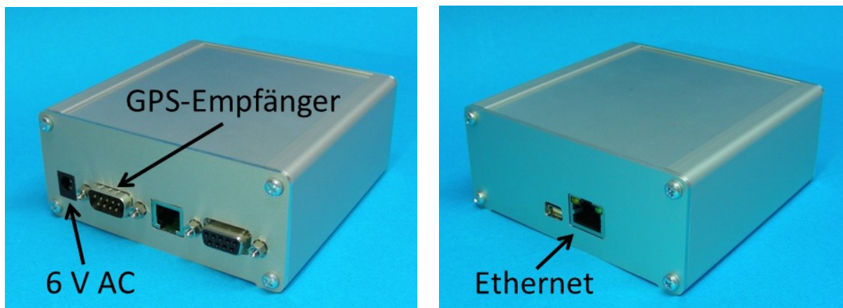
Abbildung 2: Vorderseite des Messgeräts mit Spannungsversorgung und Anschluss für den GPS-Empfänger (Variante -fhgps) im linken Bild und Rückseite mit Ethernet im rechten Bild
